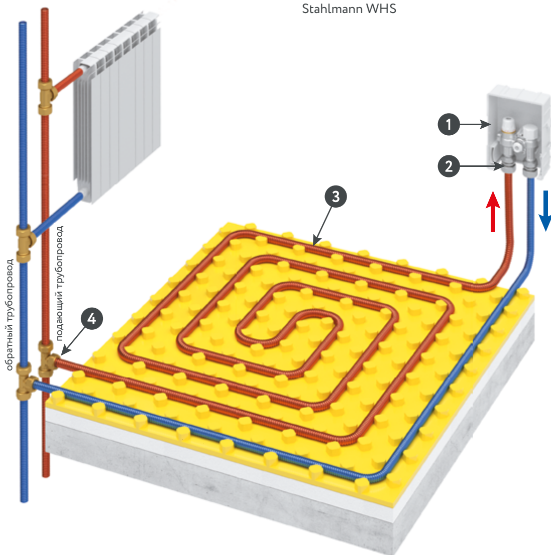
Схема подключения комплекта Stahlmann WHS
